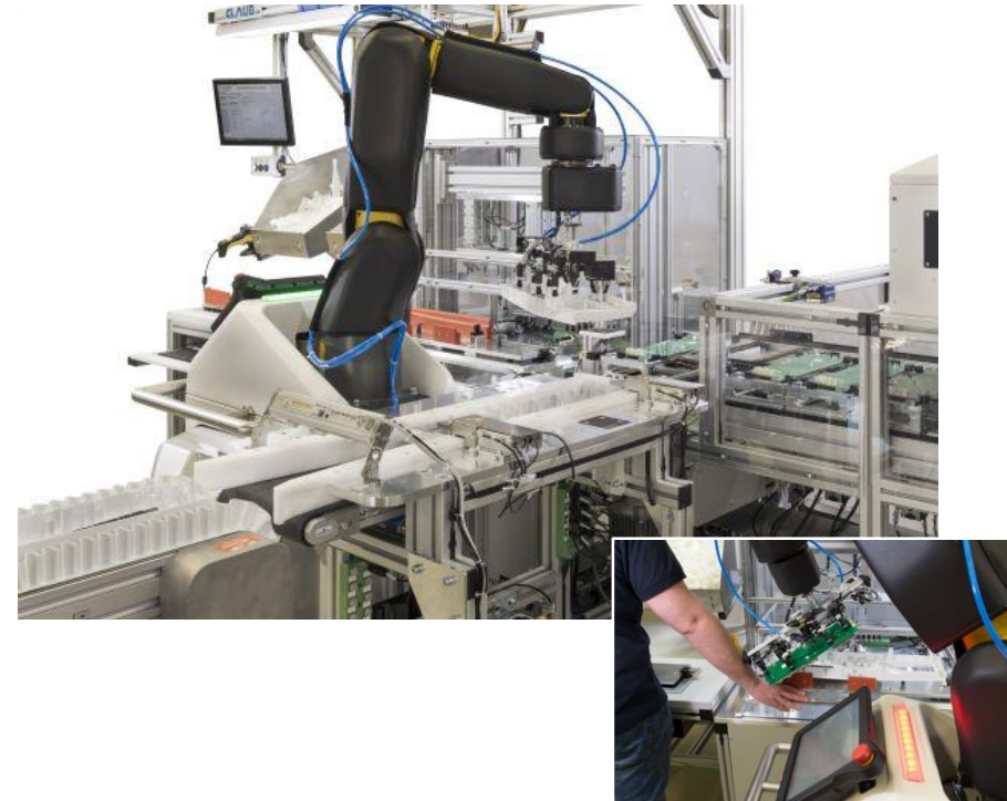
Baugruppenmontage von Waschmaschinenblenden
