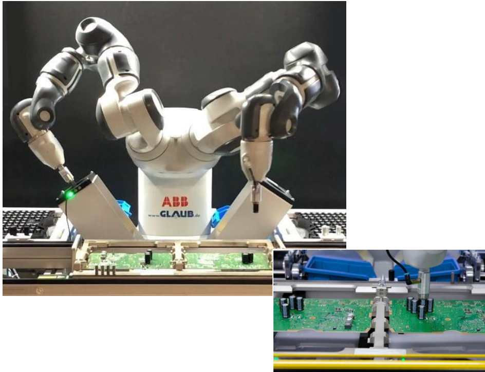
THT-Bestückung von Leiterplatten
